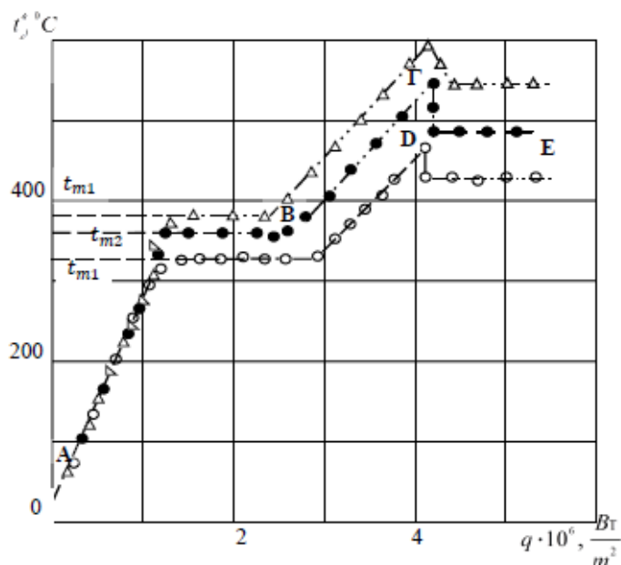
Рис.1. Характер изменения температуры внутренней стенки в зависимости от потока для подъёмного движения этилбензола при \rho\omega = 2500 \frac{кг}{м^2} \cdot с . 1 – 4.0; 2 – 5.0; 3 – 6.0 МПа
